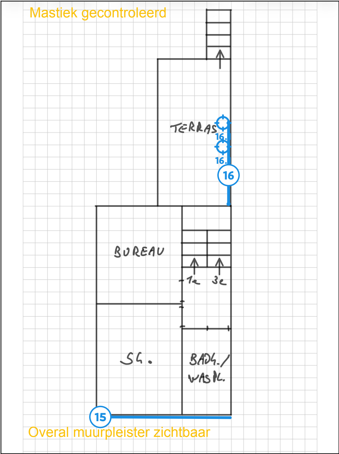
Legende van plan 2.5: 2de verdiep
